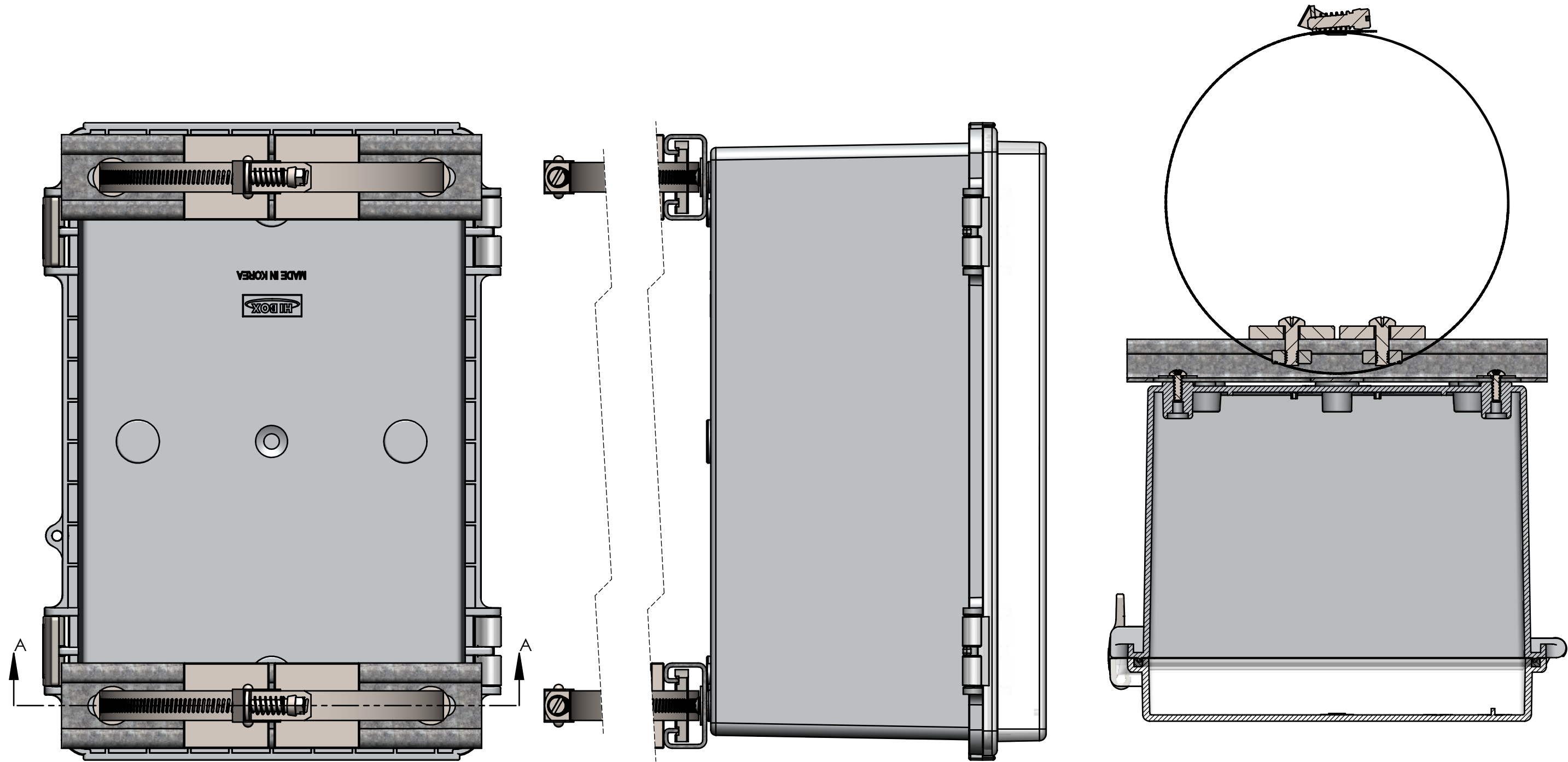
SECTION A-A
