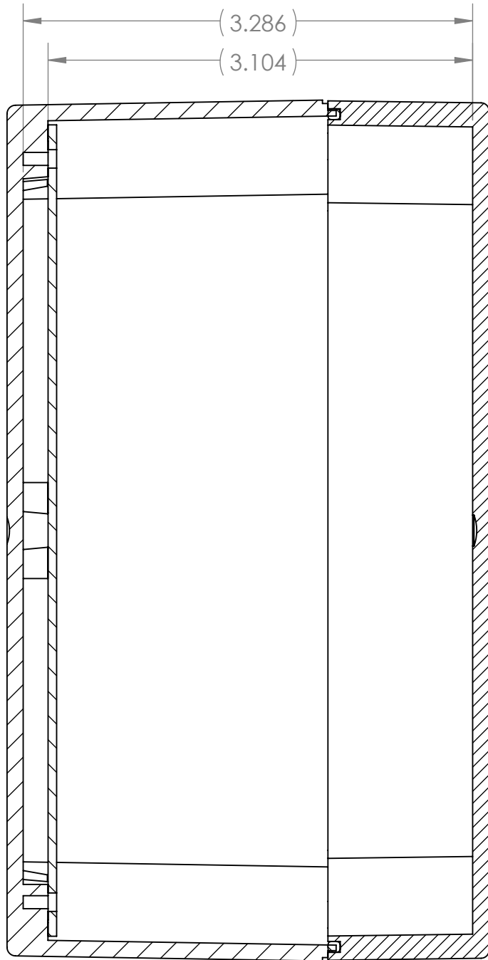
SECTION A-A
