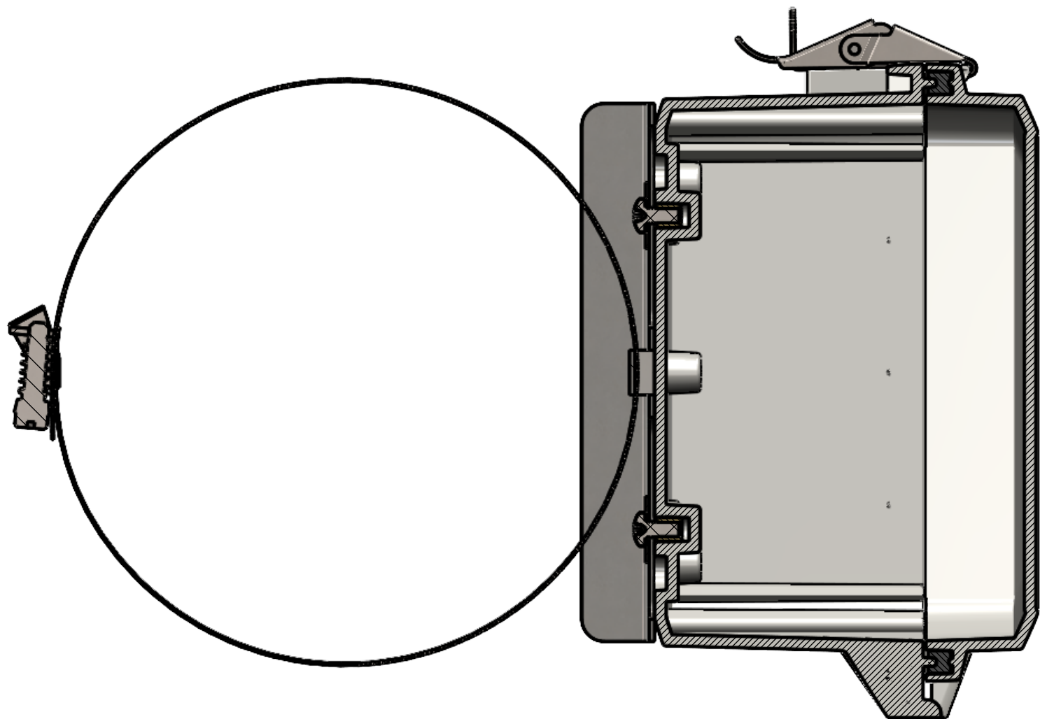
SECTION A-A
