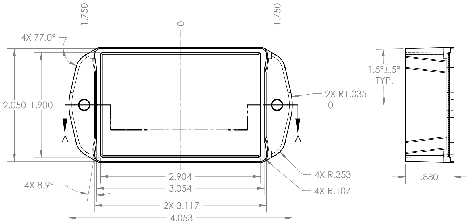
SECTION A-A
