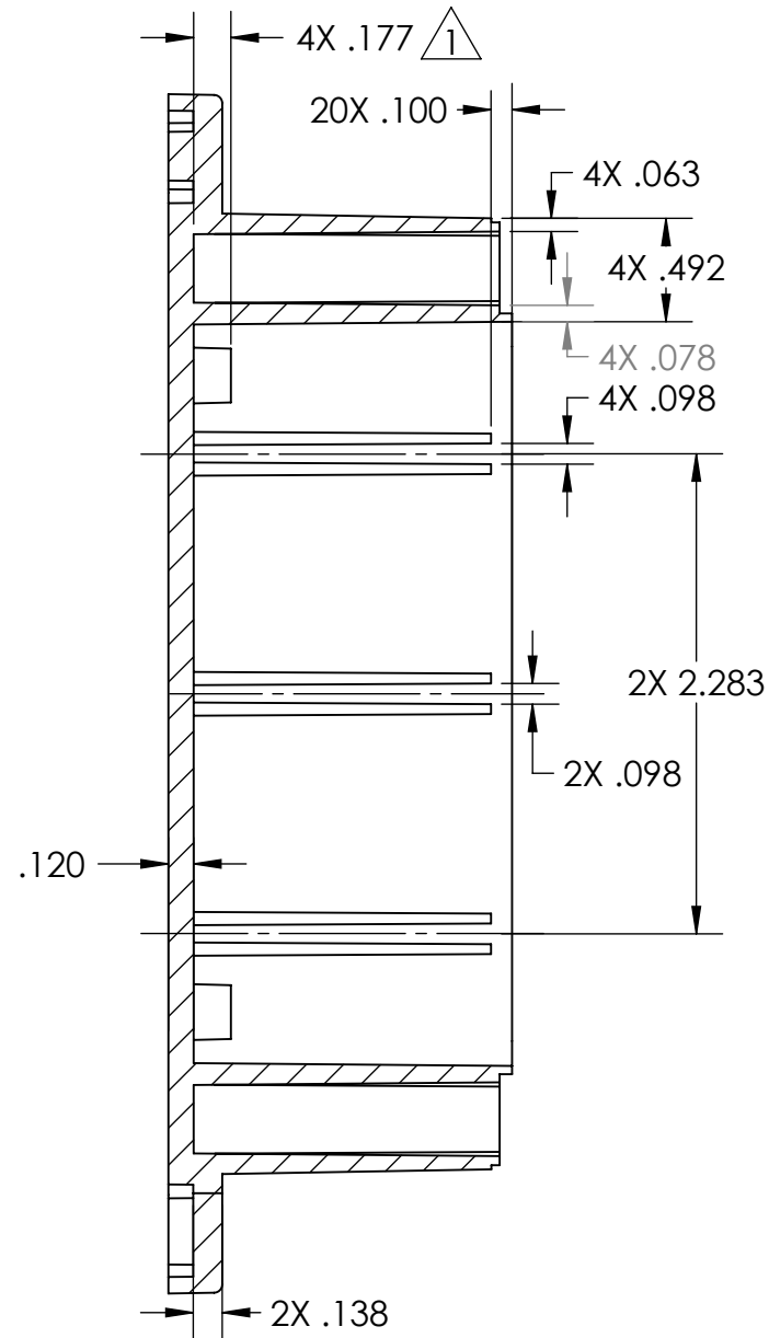
SECTION A-A
