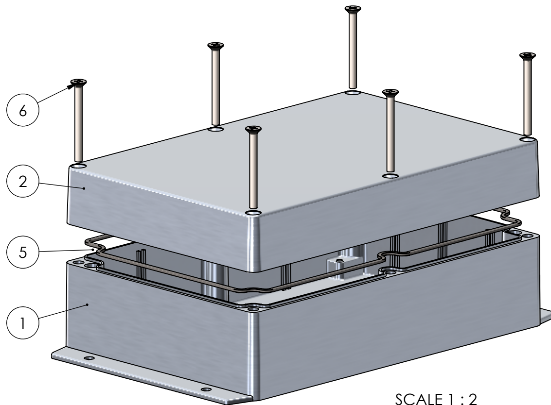
SCALE 1 : 2
