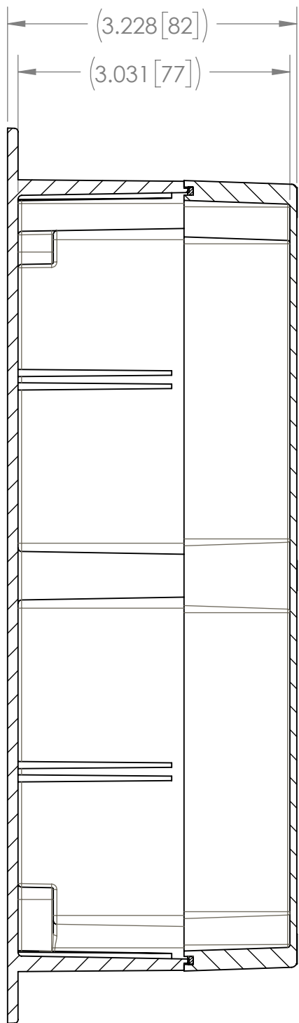
SECTION A-A
