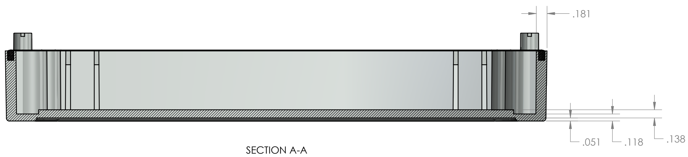
SECTION A-A
